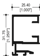
7106 CERCO TRASLAPE
