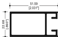
7105 CERCO CHAPA
