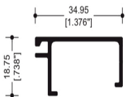
28939 JUNQUILLO
