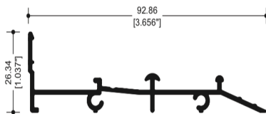
7110 RIEL CONTRAMARCO CORREDIZO
