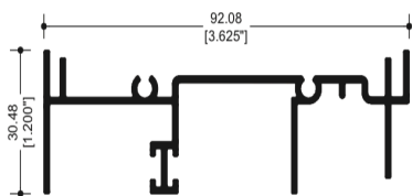
7109 CABEZAL CONTRAMARCO CORREDIZA
