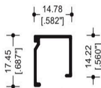
36370 JUNQUILLO
