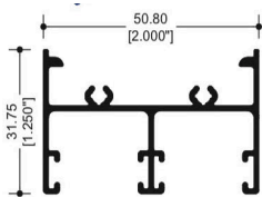
67518 CABEZAL Y JAMBA
