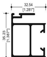
67844 CERCO TRASLAPE VENTANA
