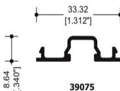
39075 TAPA BOLSA
