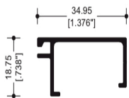
28939 JUNQUILLO
